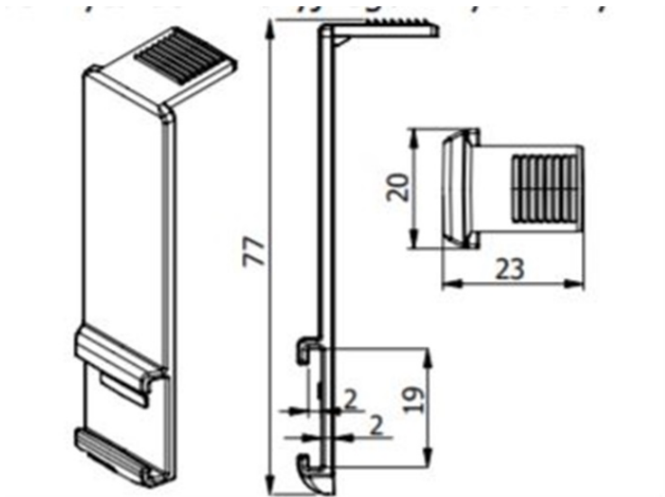
Wieszak nastawny do okien z wywietrznikiem.
